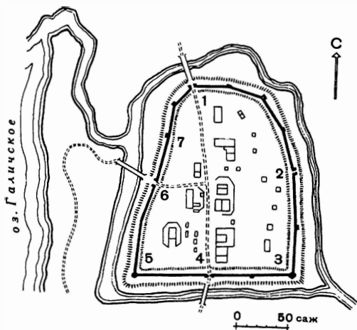
Галич. План укреплений второй половины XV в. (По чертежу начала XVIII в. и описи 1628 г.)
